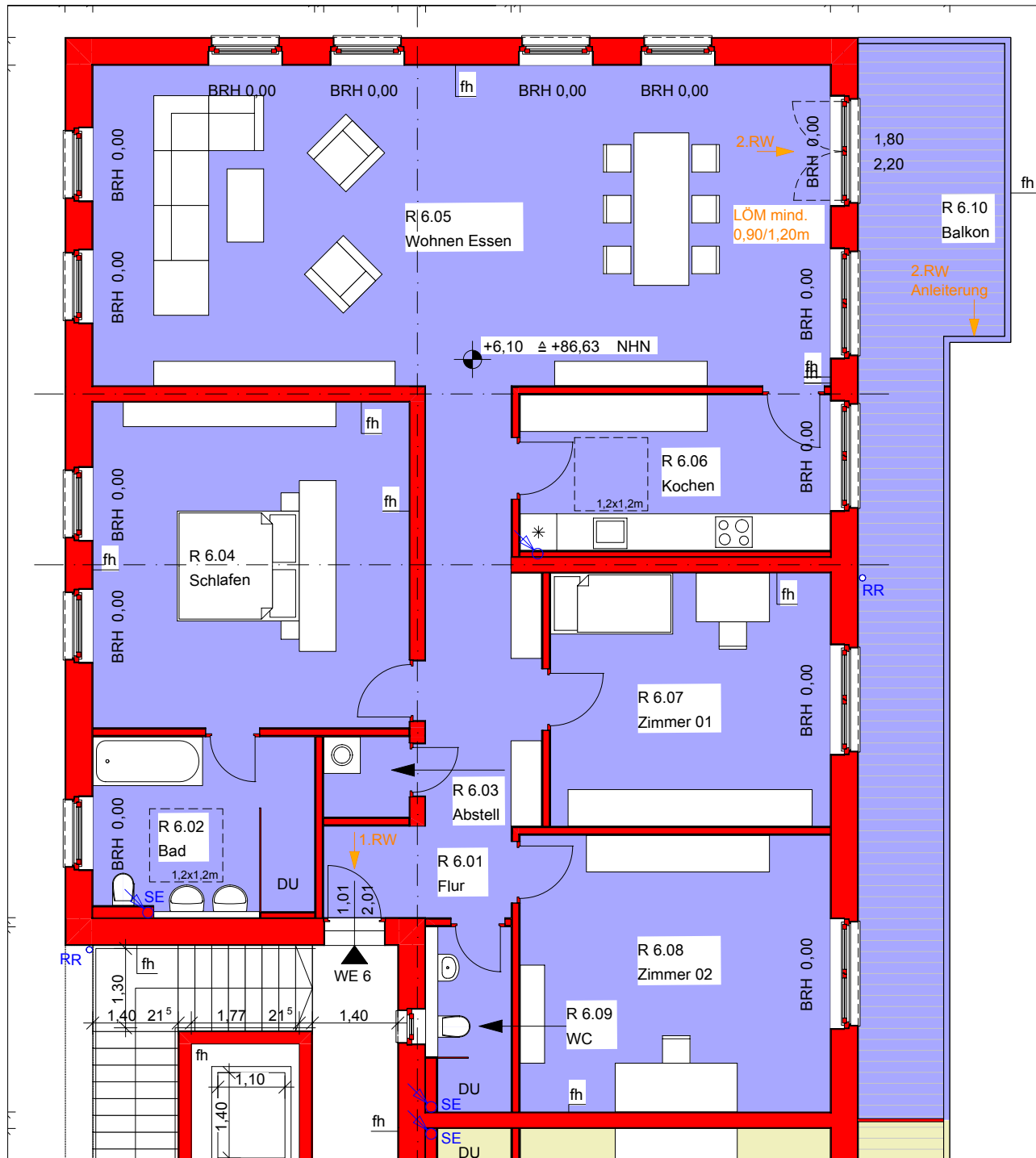
Grundriss Wohnung 6 DG
